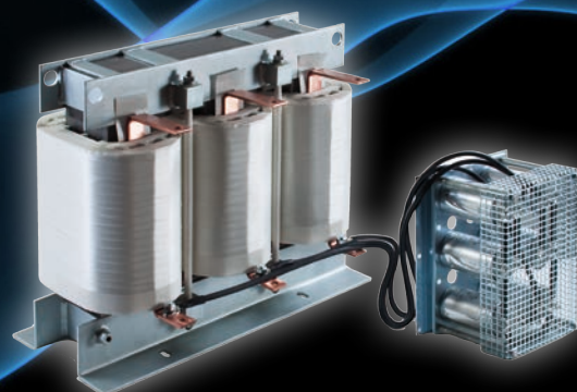
Sinusfilter över 180 A levereras med en separat kondensator-modul för ett enklare och flexibla montage.
