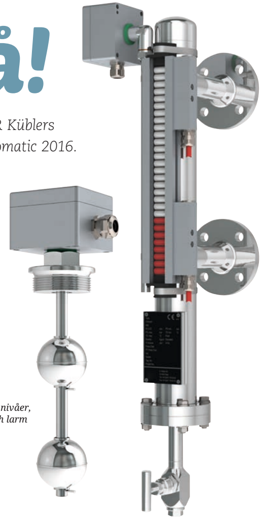
Nivåindikator som indikerar nivån lokalt och/eller med elektrisk utsignal
